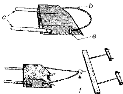
B: Simple earth scoop.
